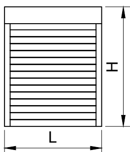
PA 39 Profil roletowy aluminiowy wypełniony pianką poliuretanową, bezfreonową
